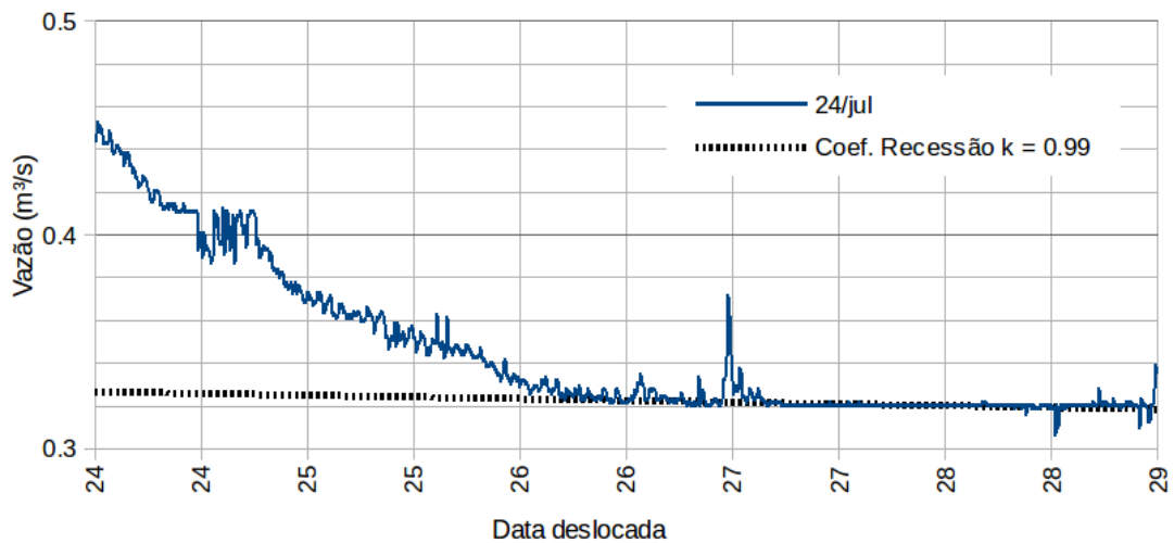
Figura 39 – Curvas de recesso da bacia 9 “Rio João Gualberto” – k = 0.99
