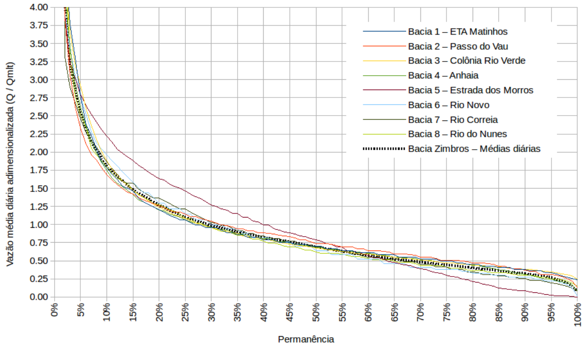
Figura 27 – Curvas de permanência de vazões médias diárias adimensionalizadas
