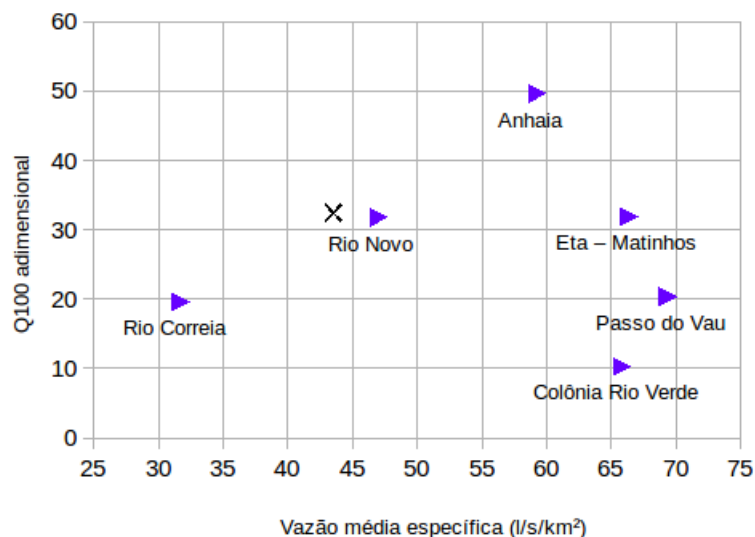
Figura 47 – Vazões Q100 adimensionalizadas ( Q_{100}/Q_{mlt} ) em função da vazão média específica. A marcação em “X” indica a posição da bacia de Zimbros.
