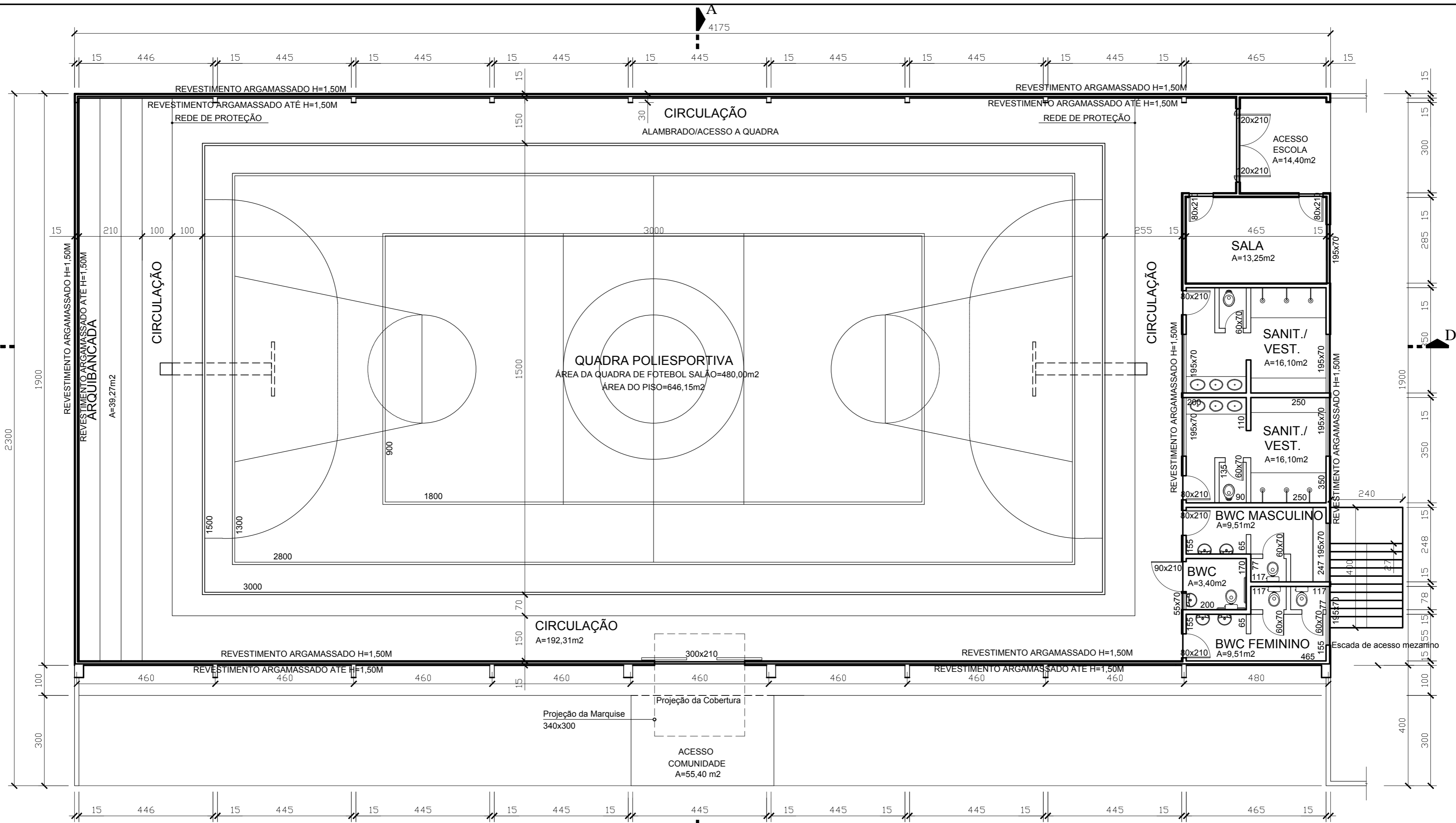
PLANTA BAIXA A= 793,85m 2 Escala 1:125
