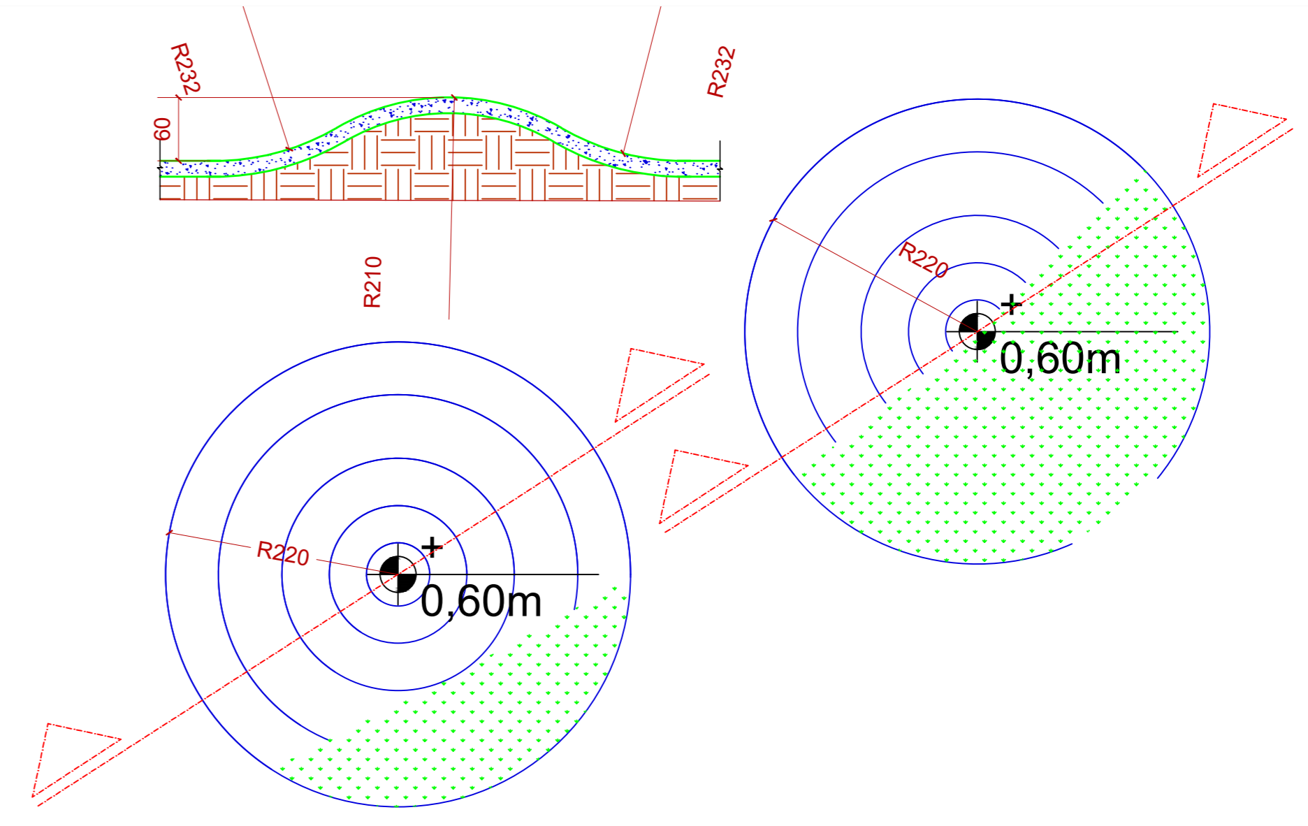
DET 06
