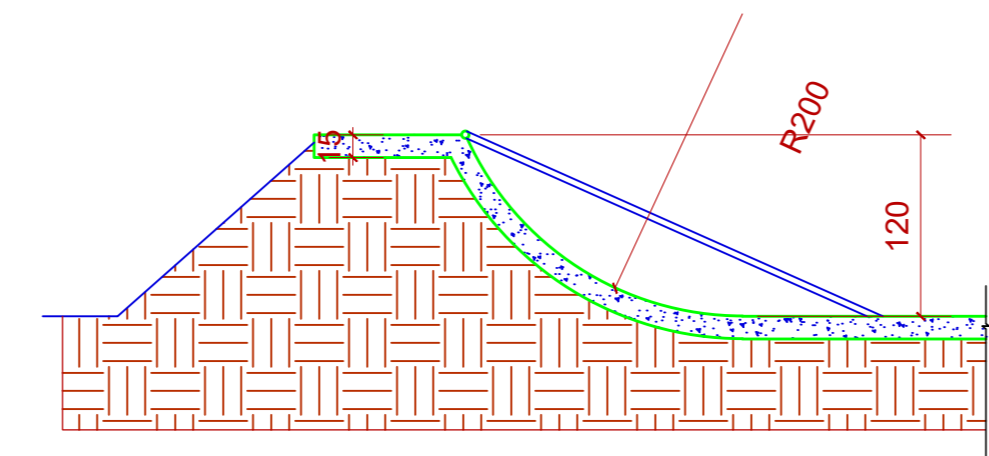
DET 05
