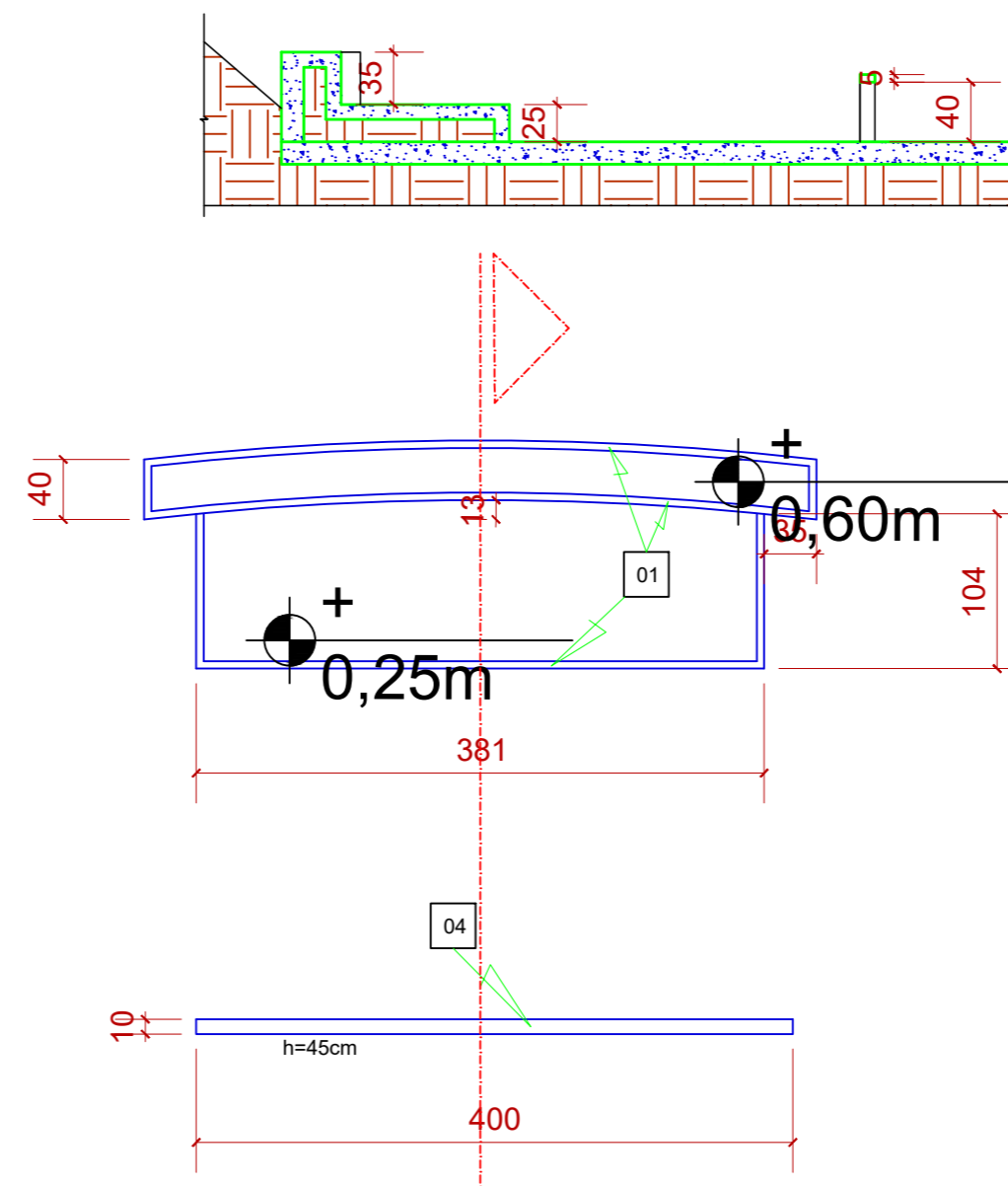
DET 10
