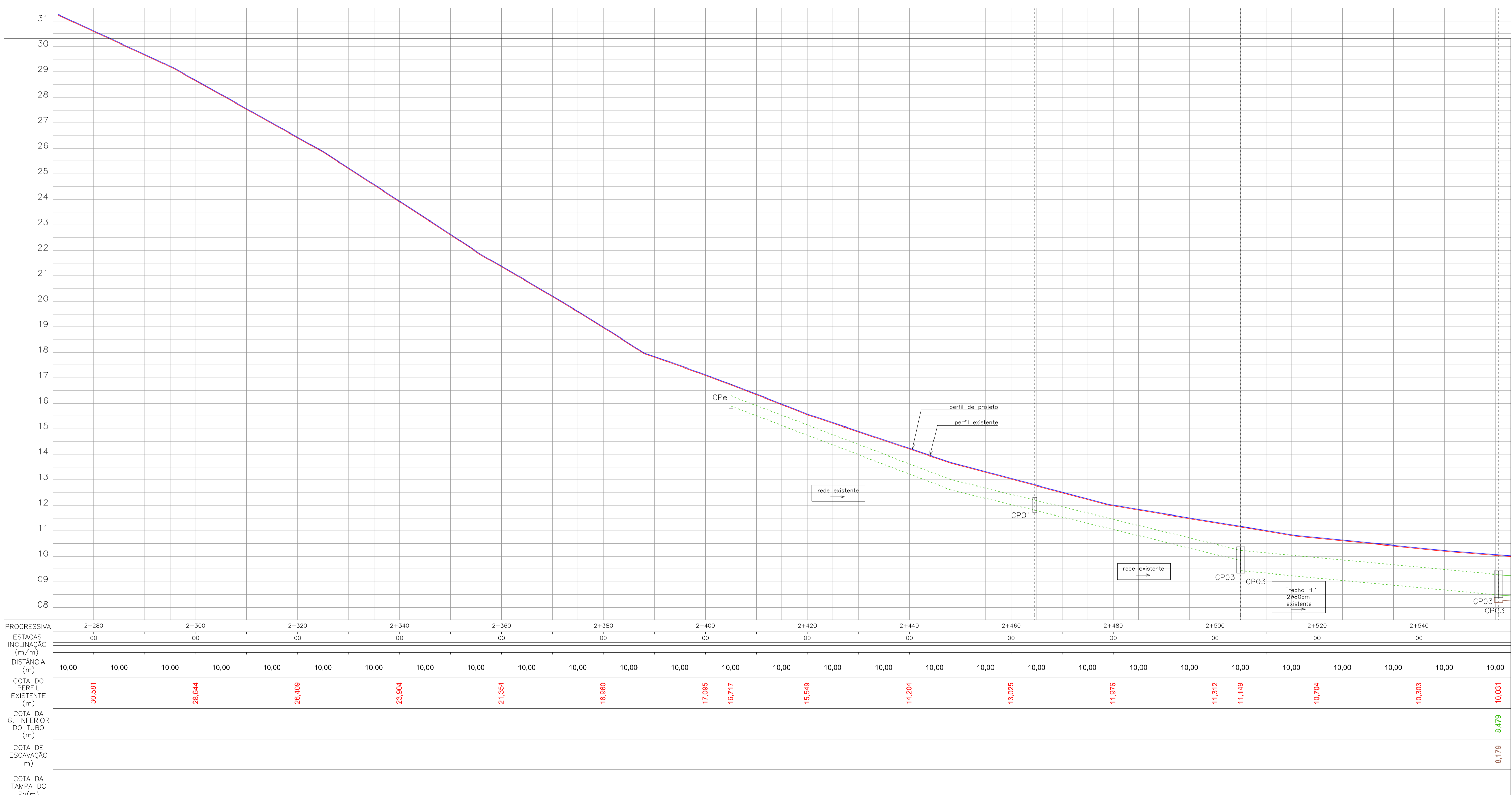
PERFIL LONGITUDINAL - ARTICULAÇÃO 09 - Rua Araçá Escala 1:500 y1:100
