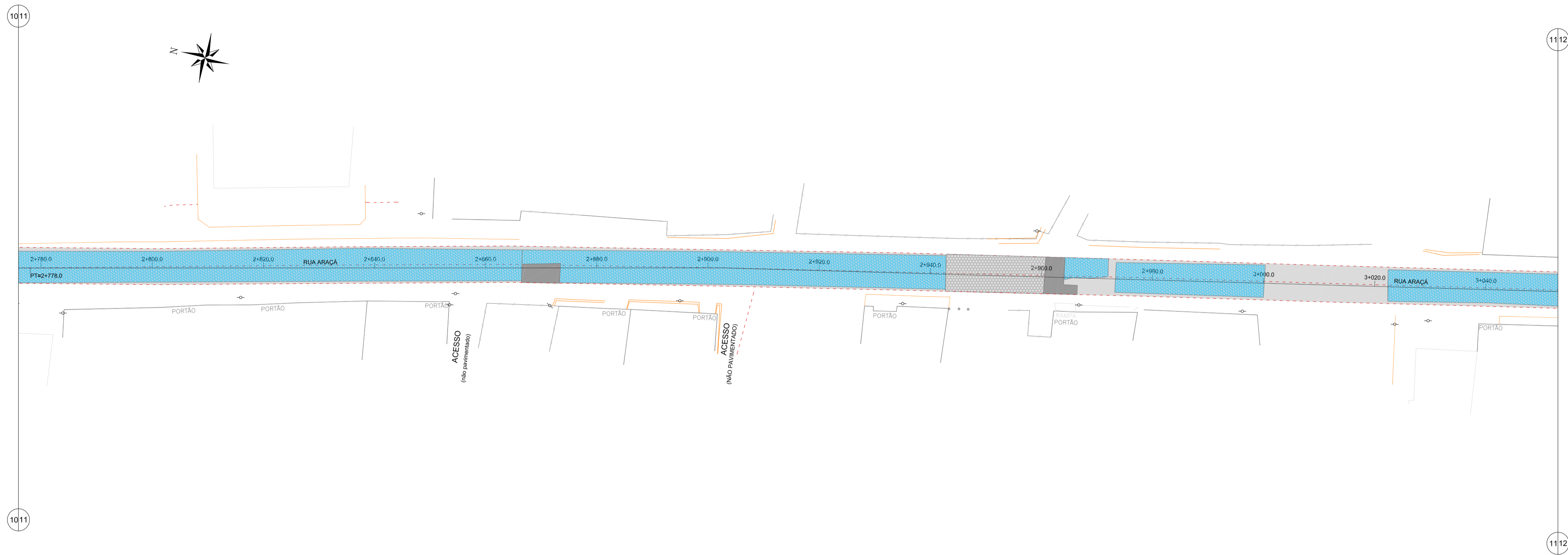
DIAGNÓSTICO DA PAVIMENTAÇÃO EXISTENTE - ARTICULAÇÃO 11 - Rua Araçá Escala 1:500
