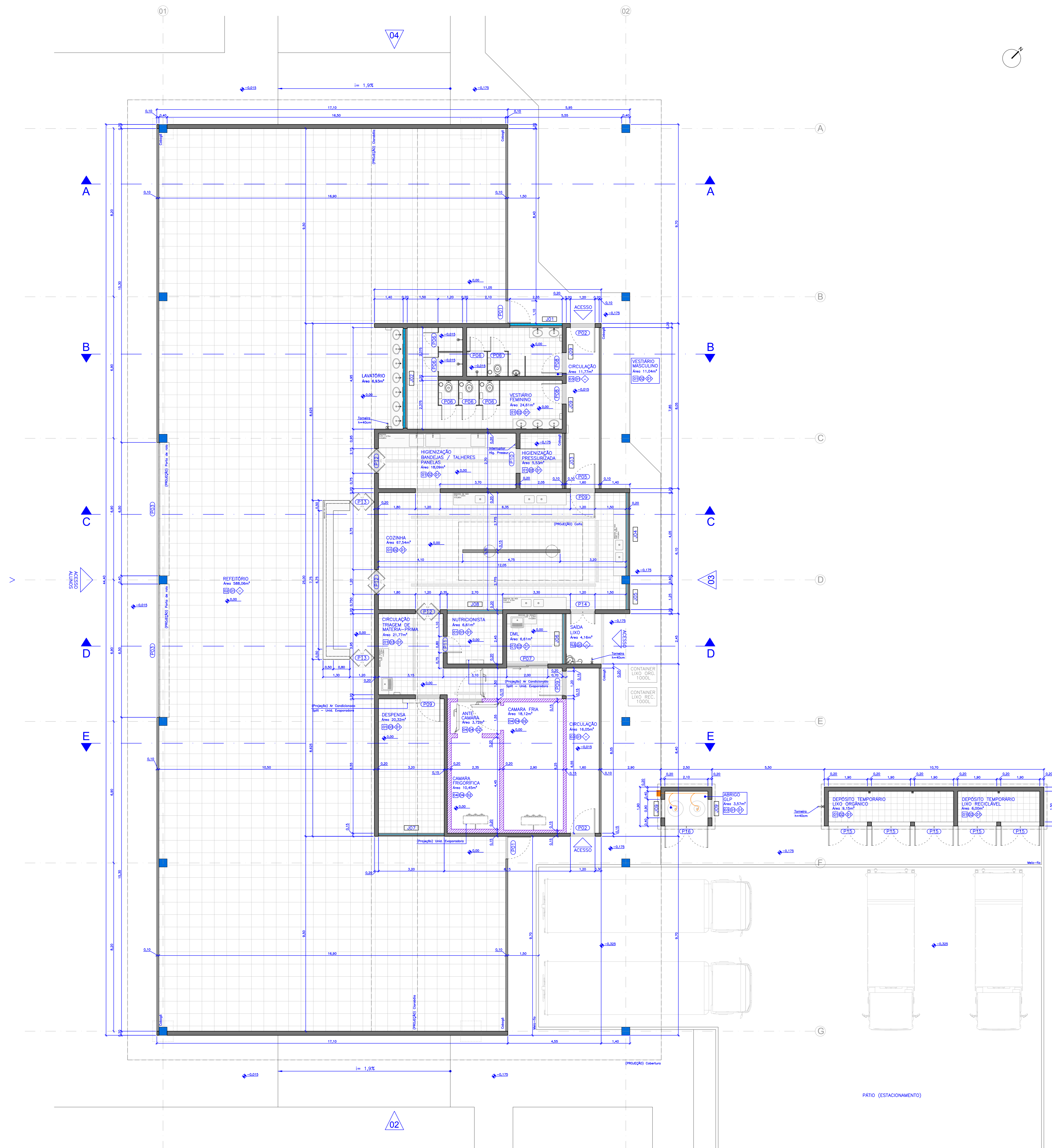
04 PLANTA BAIXA - TÉRREO (CONSTRUTIVO) Escala 1:75
