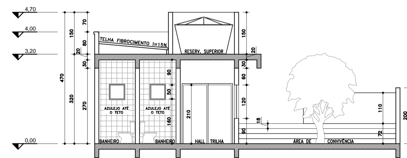
CORTE A-A ESCALA 1/75
