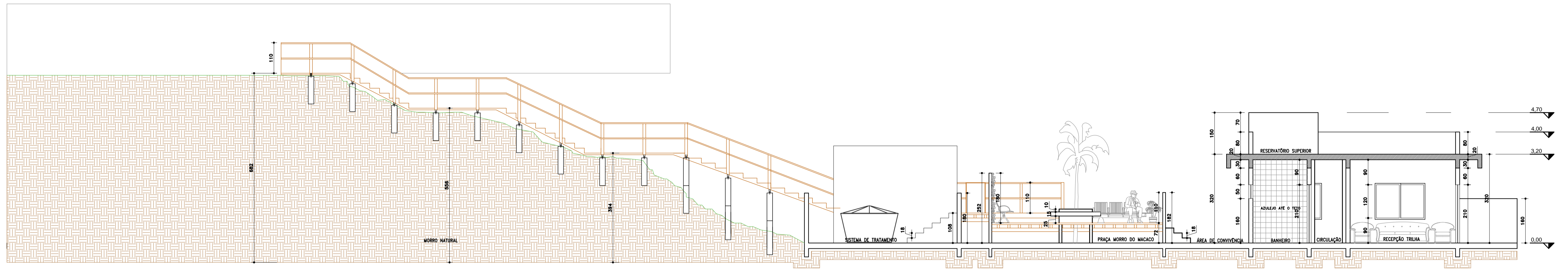
CORTE B-B ESCALA 1/75
