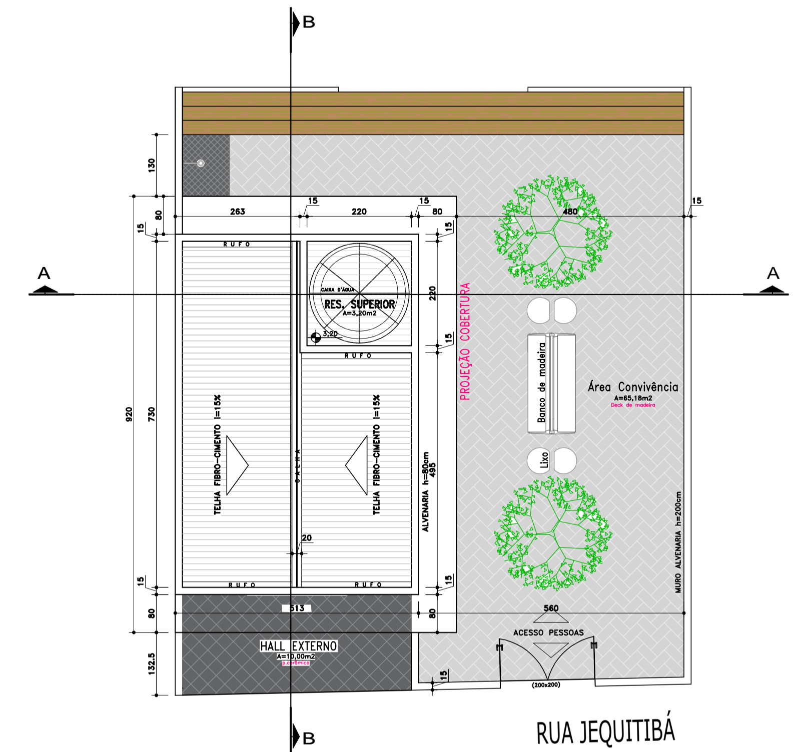
COBERTURA ESCALA 1/75
