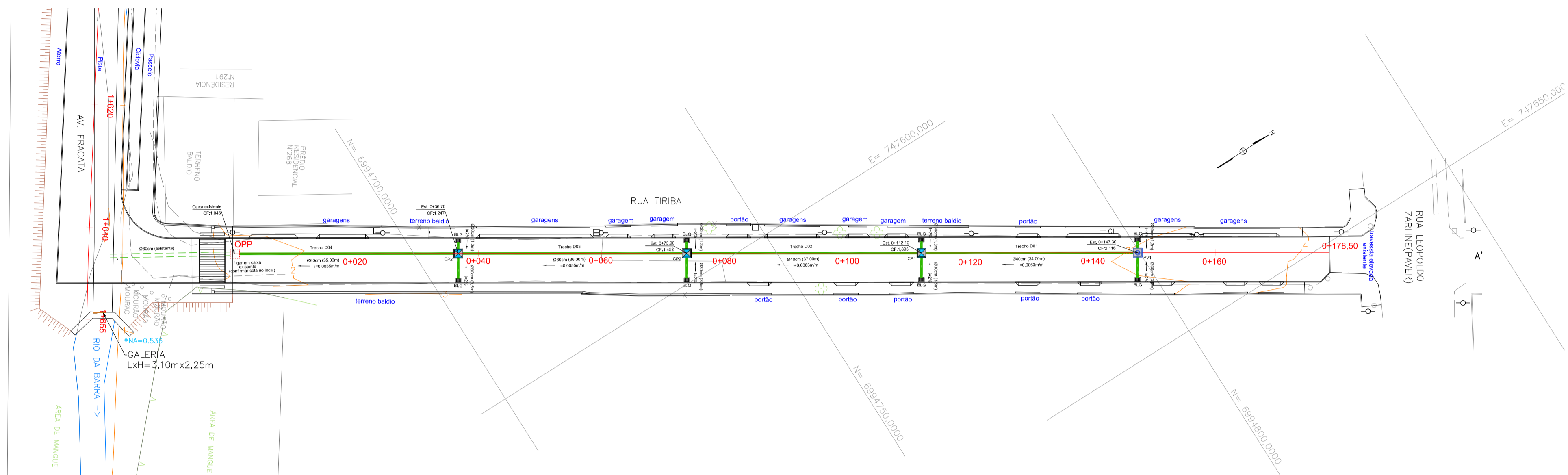
Drenagem Pluvial - Articulação 01 Escala 1:500
