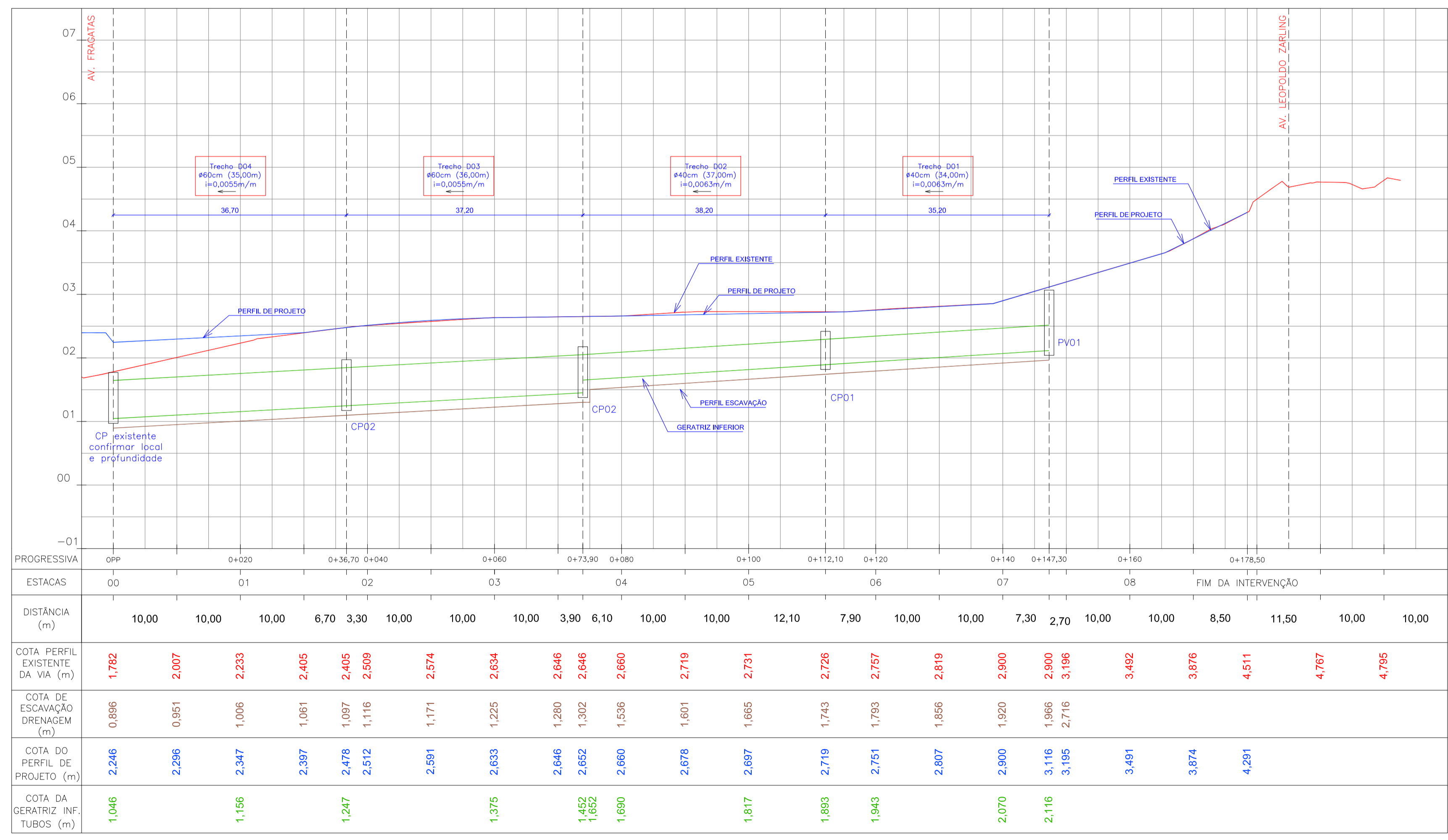
Perfil Longitudinal - Articulação 01 Escala H=1:500 / V=1:50
