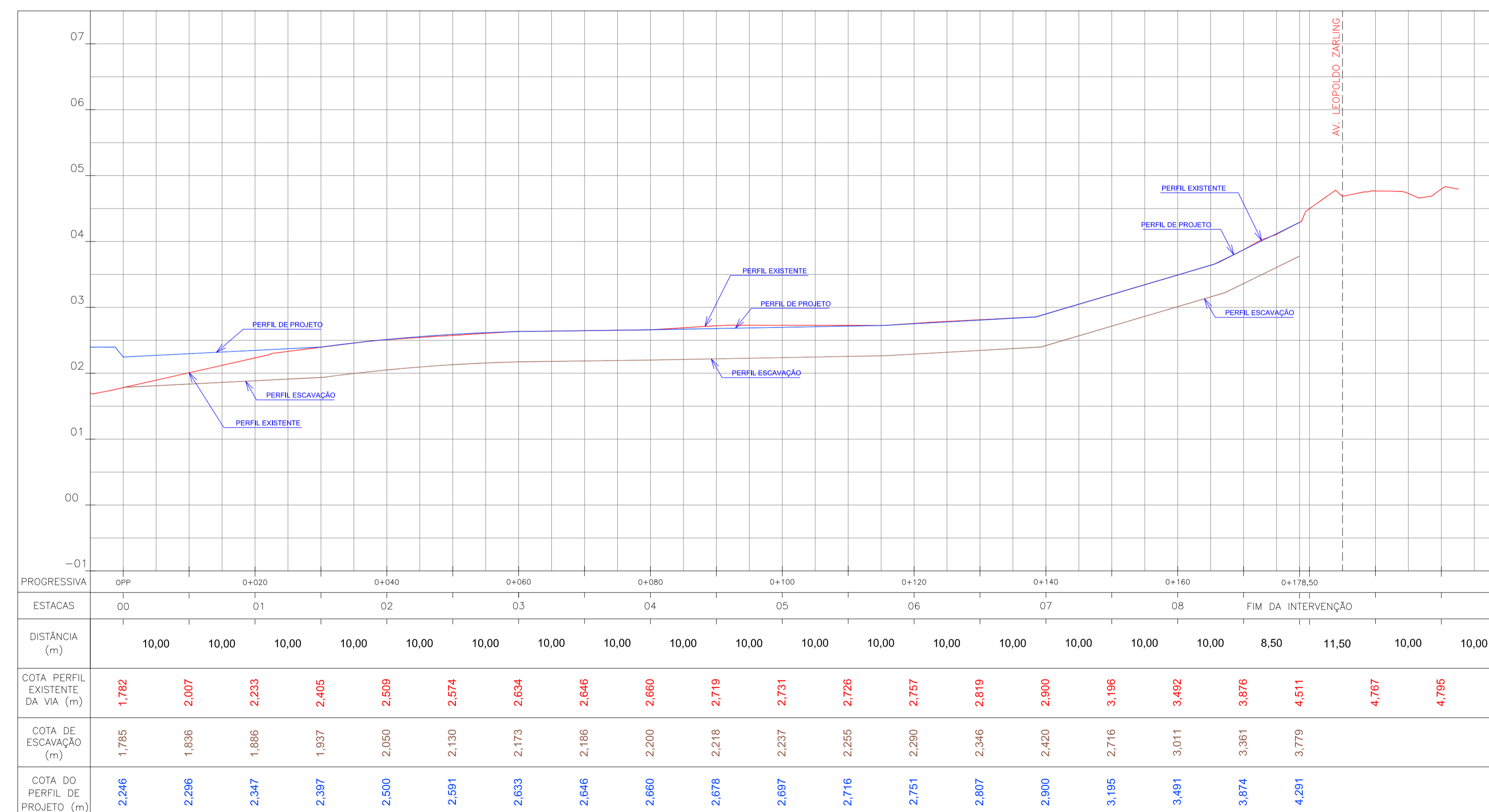
Perfil Longitudinal - Articulação 01 Escala H=1:500 / V=1:50
