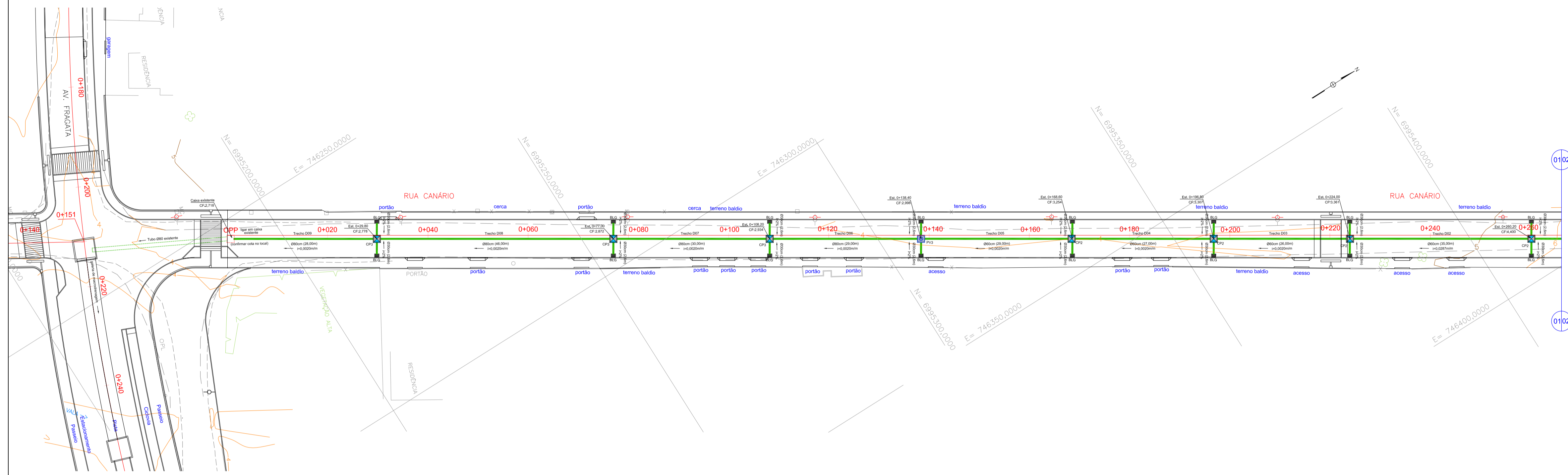
Drenagem Pluvial - Articulação 01 Escala 1:500
