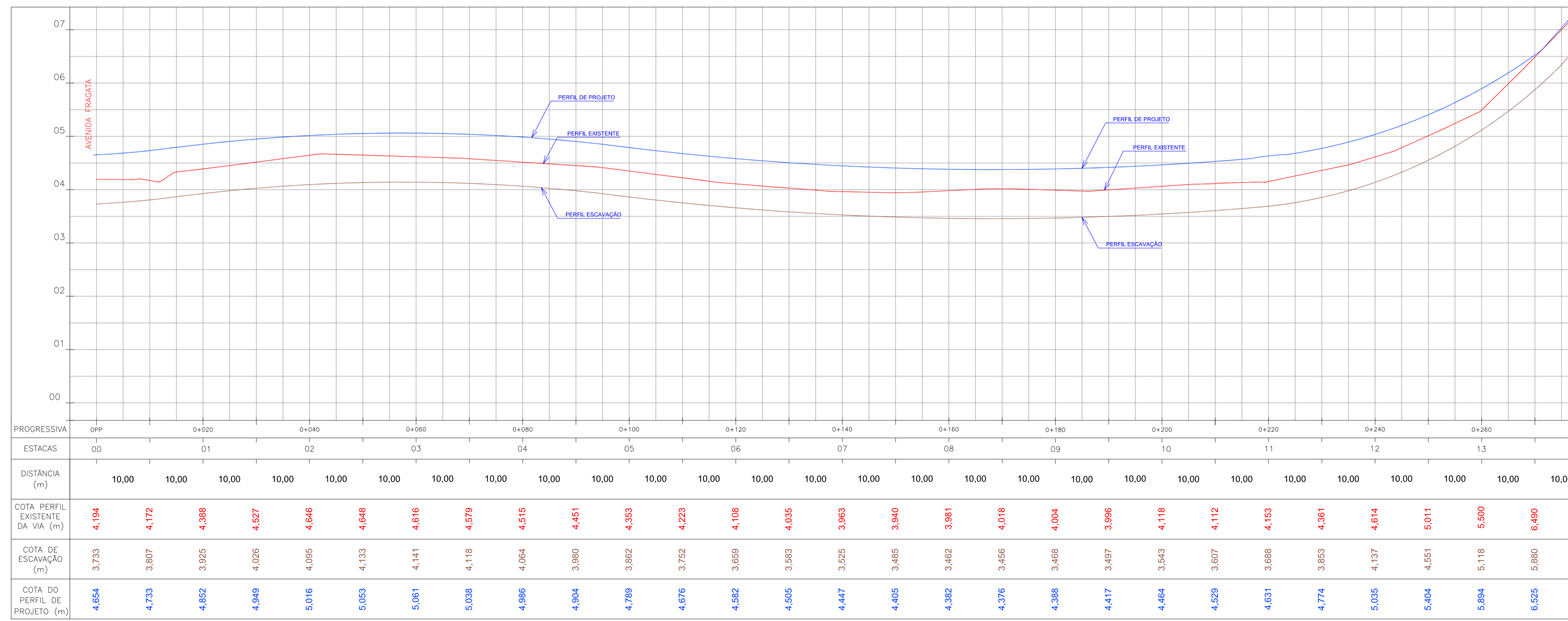
Perfil Longitudinal - Articulação 01 Escala H=1:500 / V=1:50
