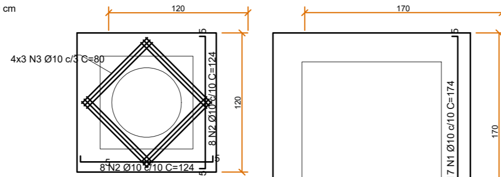
DETALHE DA TAMPA EM CONCRETO ARMADO
