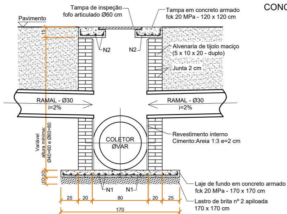
CORTE AB
