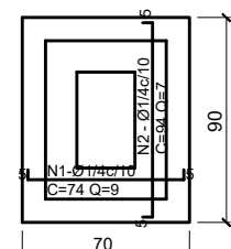
DETALHE LAJE DO FUNDO CONCRETO ESTRUTURAL
