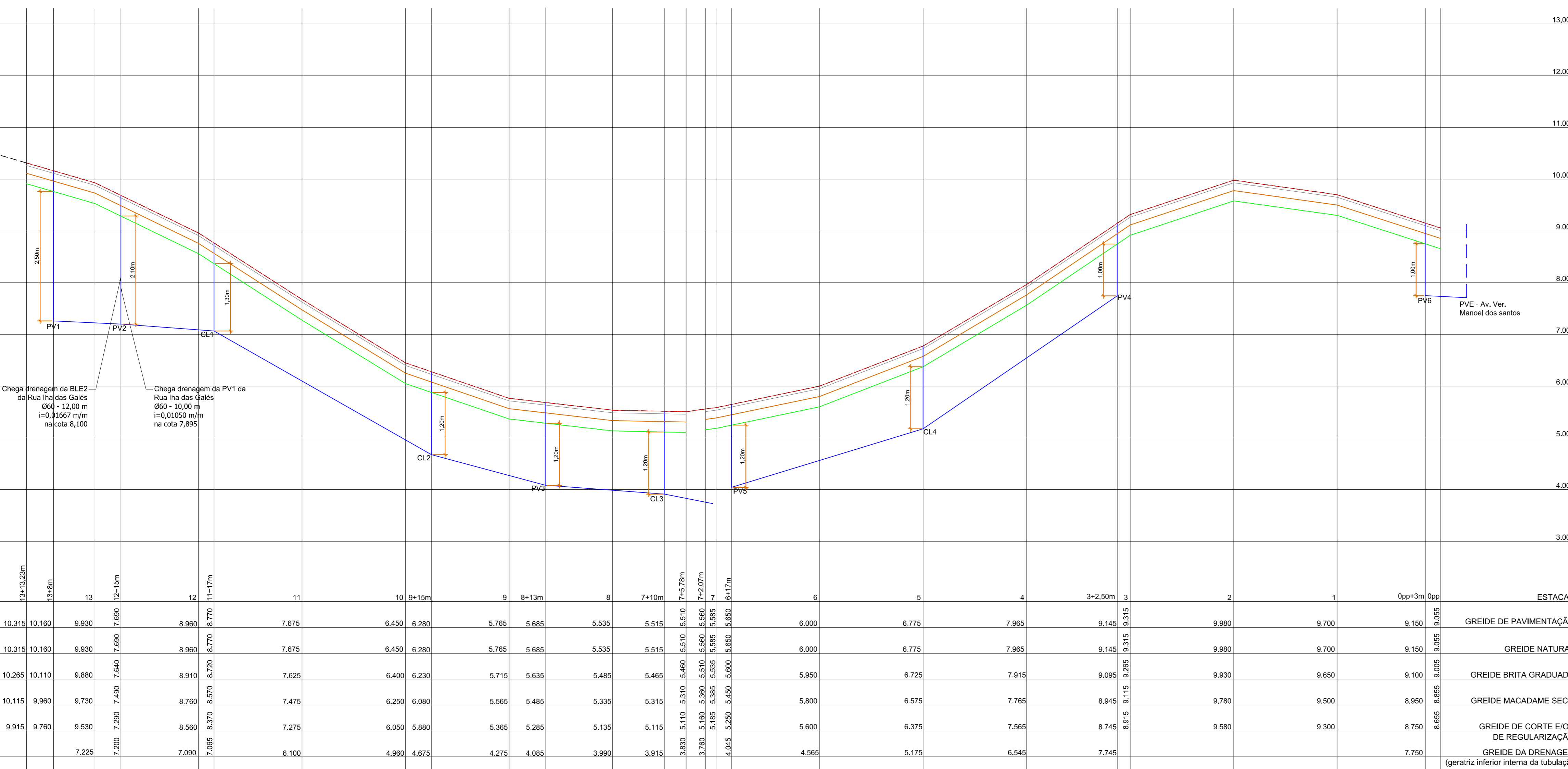
PERFIL LONGITUDINAL Rua Salmão ESCALA HORIZONTAL 1:500 ESCALA VERTICAL 1:50 ESTACAS 0pp a 13+13,23 m
