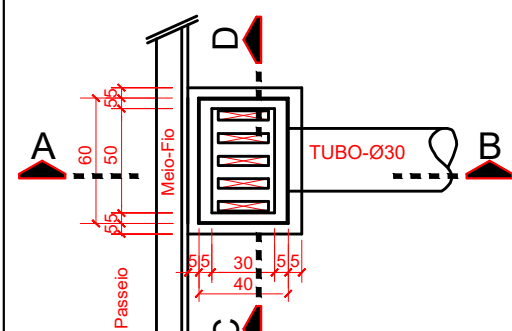
PLANTA BAIXA ETAPA - 1
