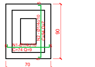
DETALHE LAJE DO FUNDO CONCRETO ESTRUTURAL
