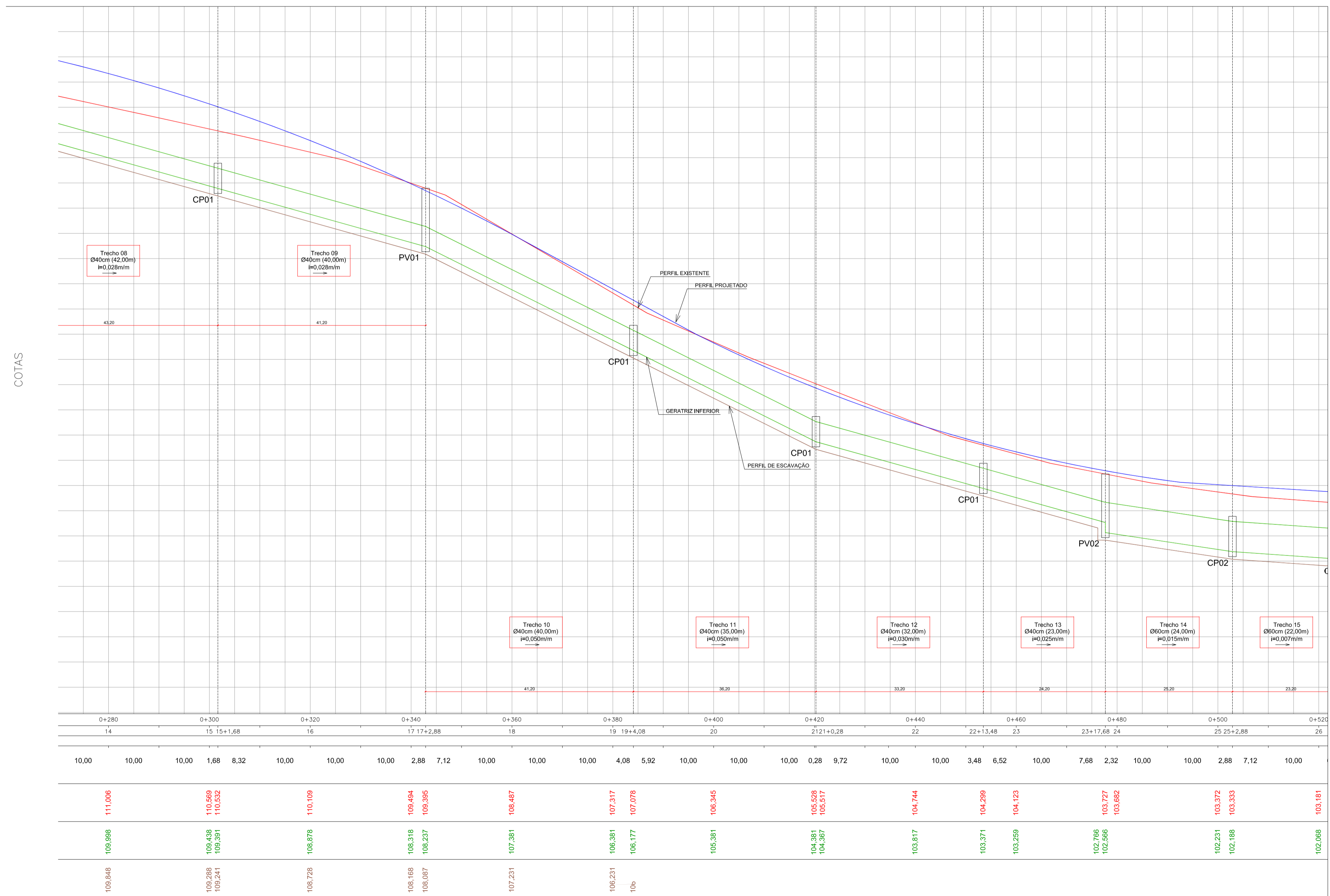
PERFIL LONGITUDINAL - Rua Martim Pescador - Articulação 02 Escala H=1:500 / V=1:50
