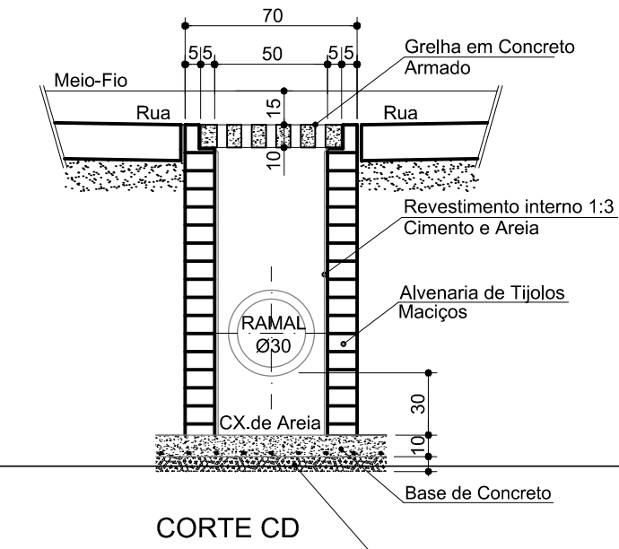
DETALHE DA GRELHA EM CONCRETO ARMADO
