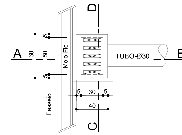
PLANTA BAIXA
