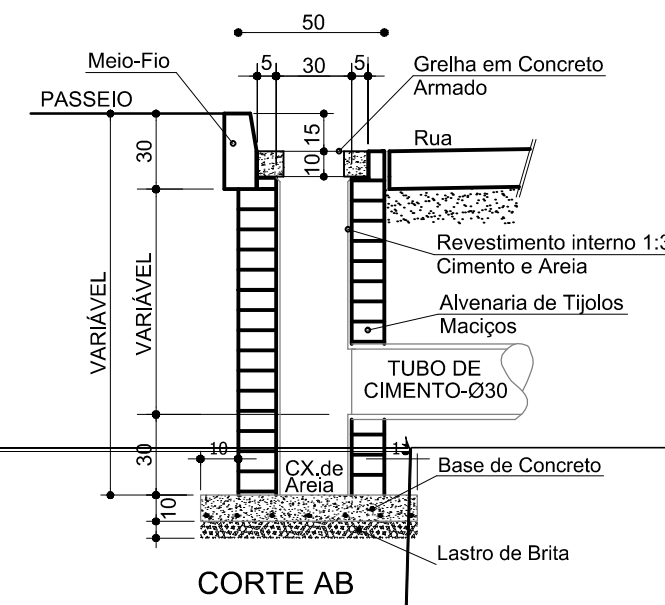
CORTE AB
