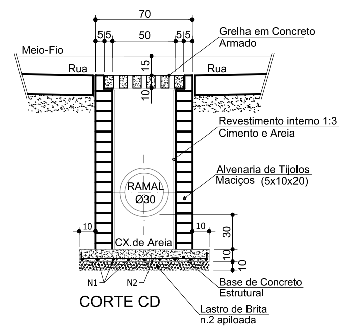
DETALHE DA GRELHA EM CONCRETO ARMADO
