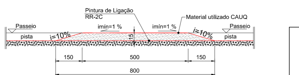
SEÇÃO AA SEM ESCALA
