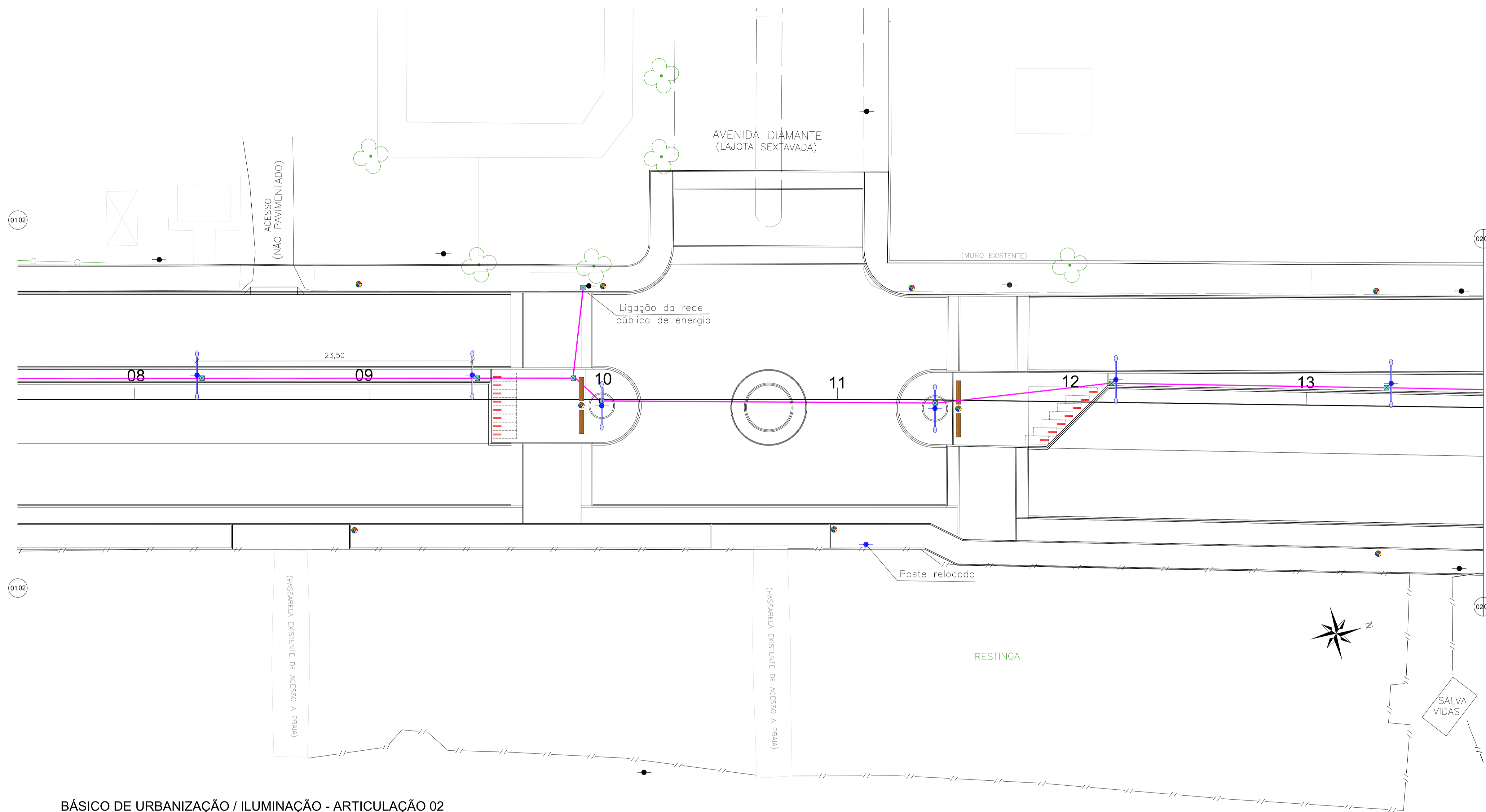
BÁSICO DE URBANIZAÇÃO / ILUMINAÇÃO - ARTICULAÇÃO 02 ESCALA 1:200
