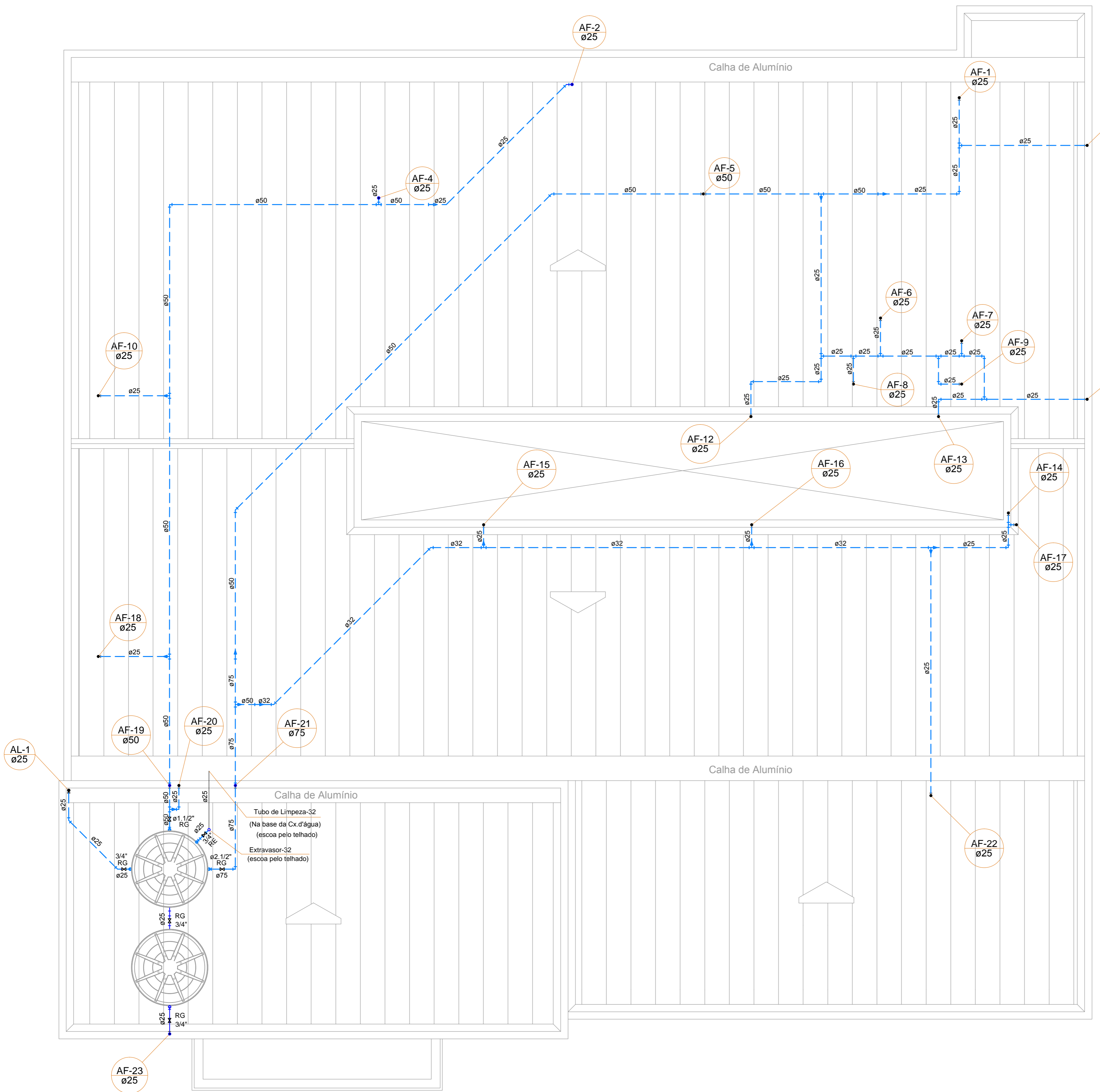
PLANTA DE DISTRIBUIÇÃO DE ÁGUA FRIA NA COBERTURA ESCALA 1:50
