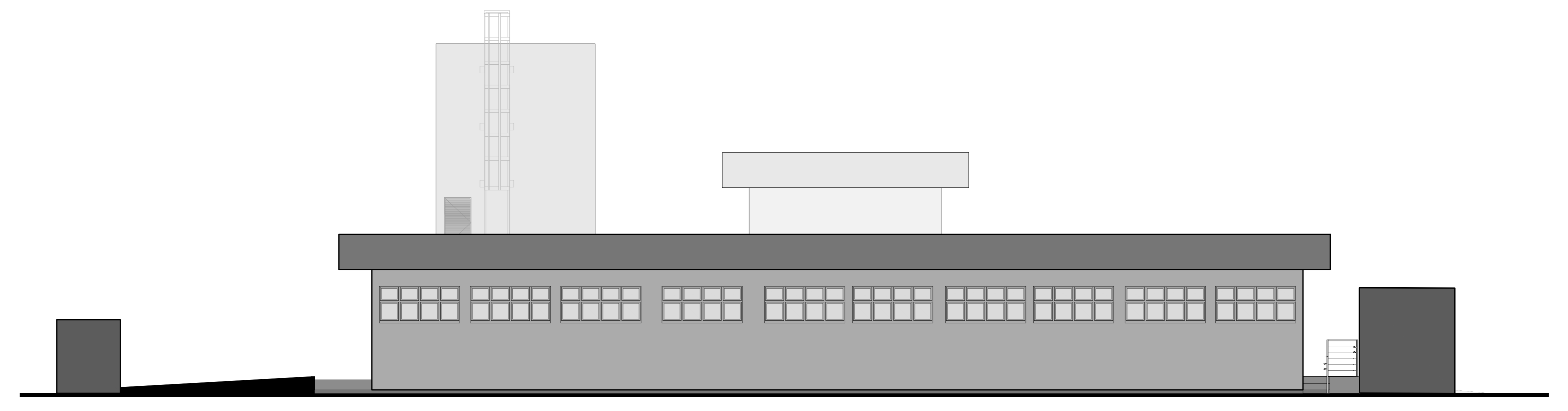
16 ELEVACÃO 04 Escala 1:75
