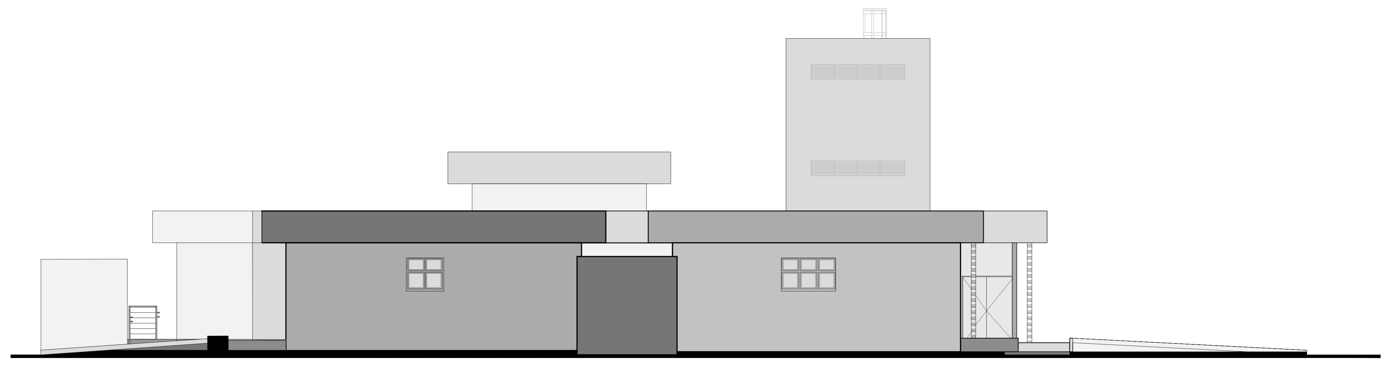
15 ELEVACÃO 03 Escala 1:75
