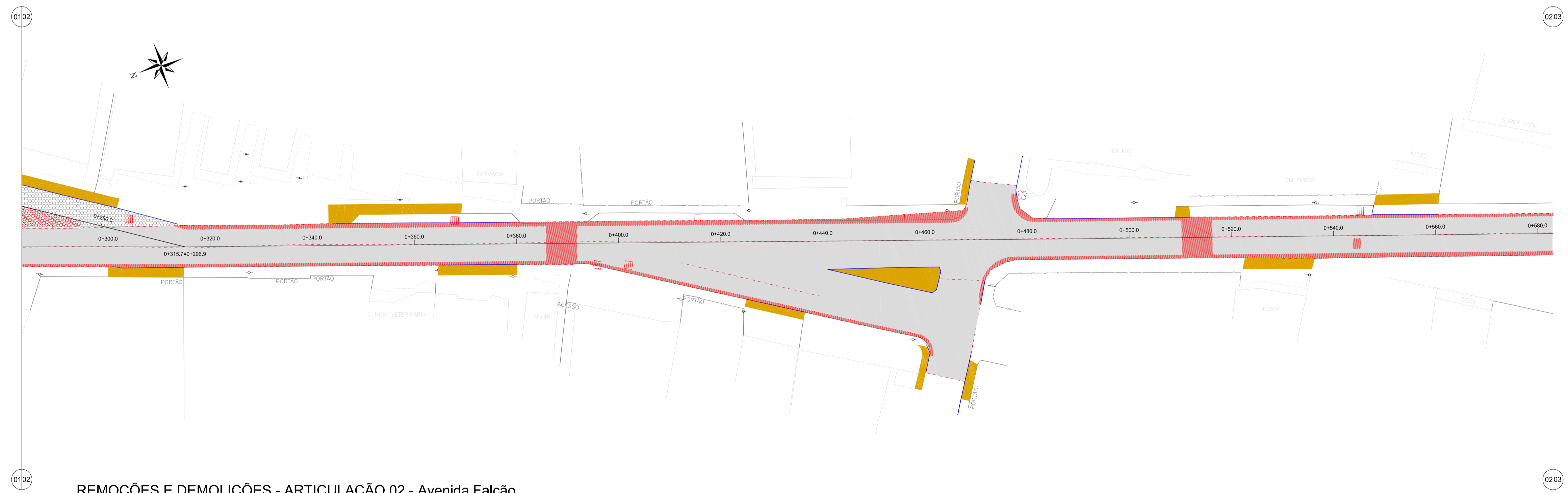
REMOÇÕES E DEMOLIÇÕES - ARTICULAÇÃO 02 - Avenida Falcão Escala 1:500
