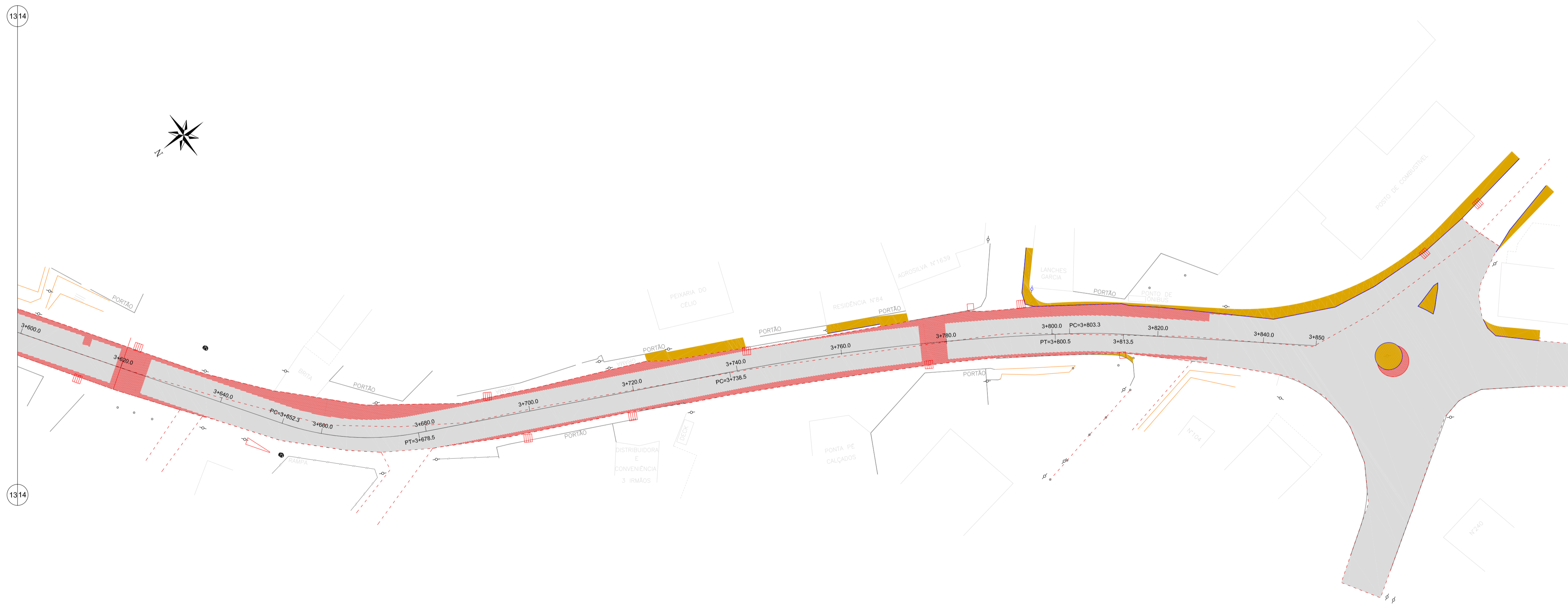
REMOÇÕES E DEMOLIÇÕES - ARTICULAÇÃO 14 - Rua Araçá Escala 1:500
