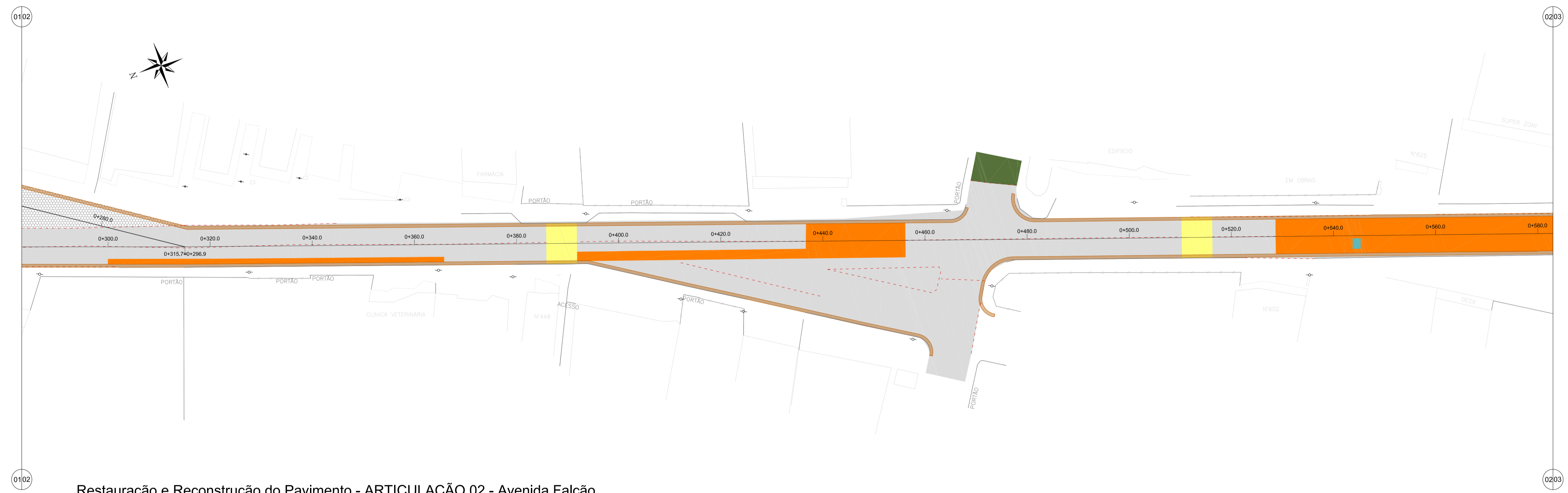
Restauração e Reconstrução do Pavimento - ARTICULAÇÃO 02 - Avenida Falcão Escala 1:500
