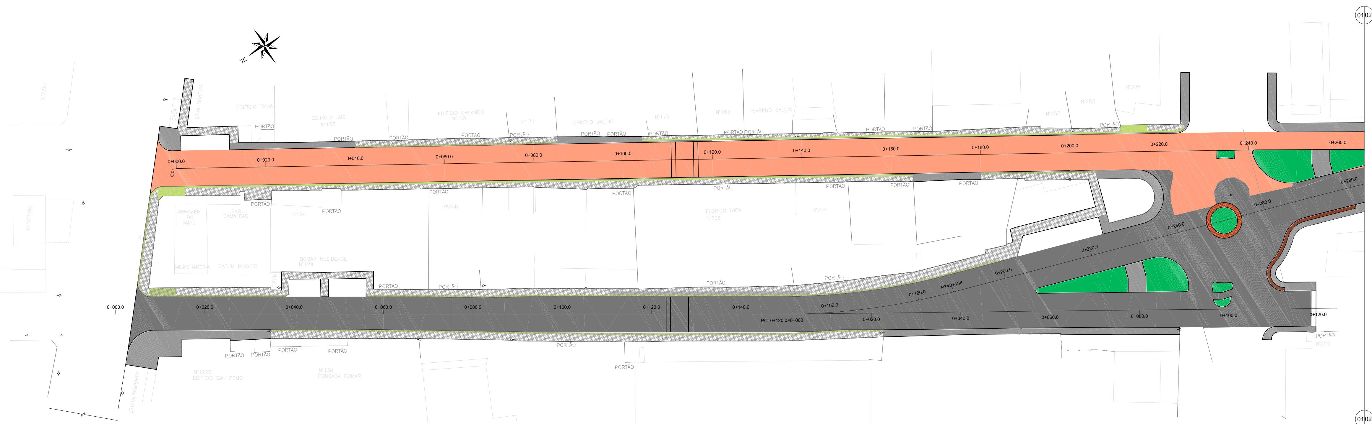
Restauração e Reconstrução do Pavimento - ARTICULAÇÃO 01 - Rua Colibri e Avenida Falcão Escala 1:500
