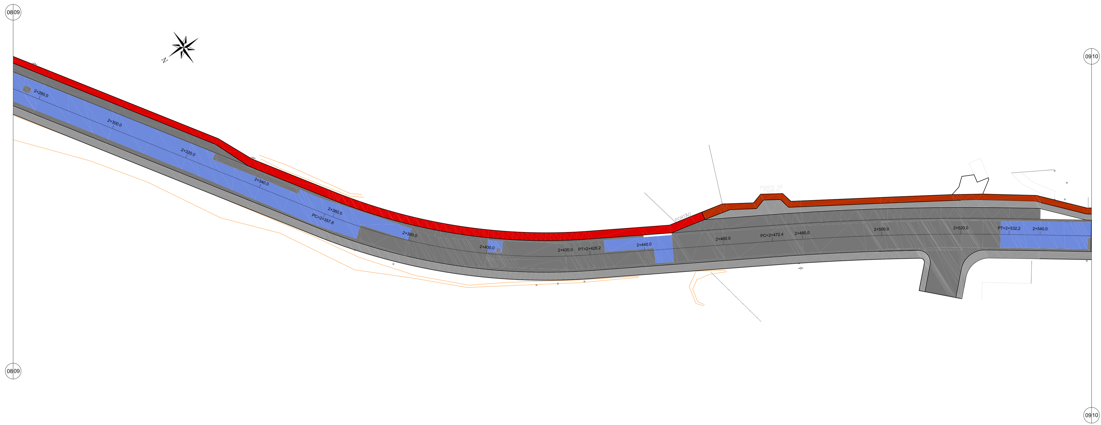
Restauração e Reconstrução do Pavimento - ARTICULAÇÃO 09 - Rua Araçá Escala 1:500
