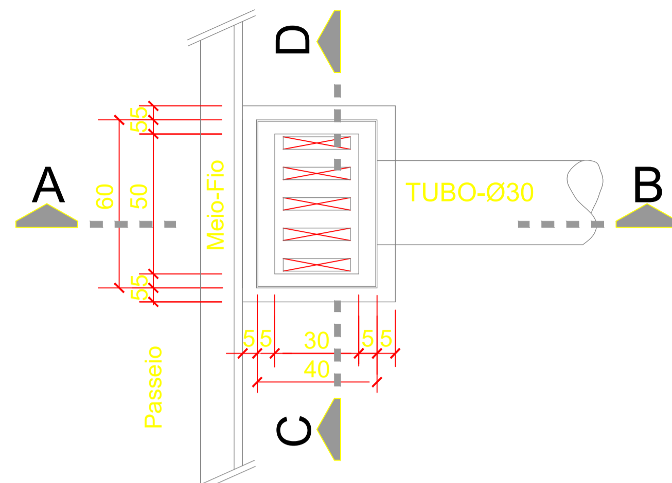
PLANTA BAIXA ETAPA - 1
