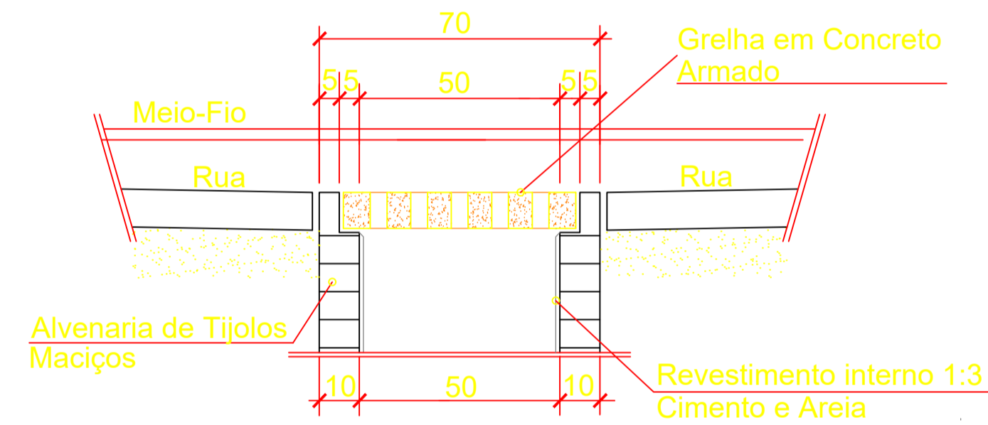
CORTE CD
