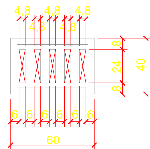
CORTE AB
