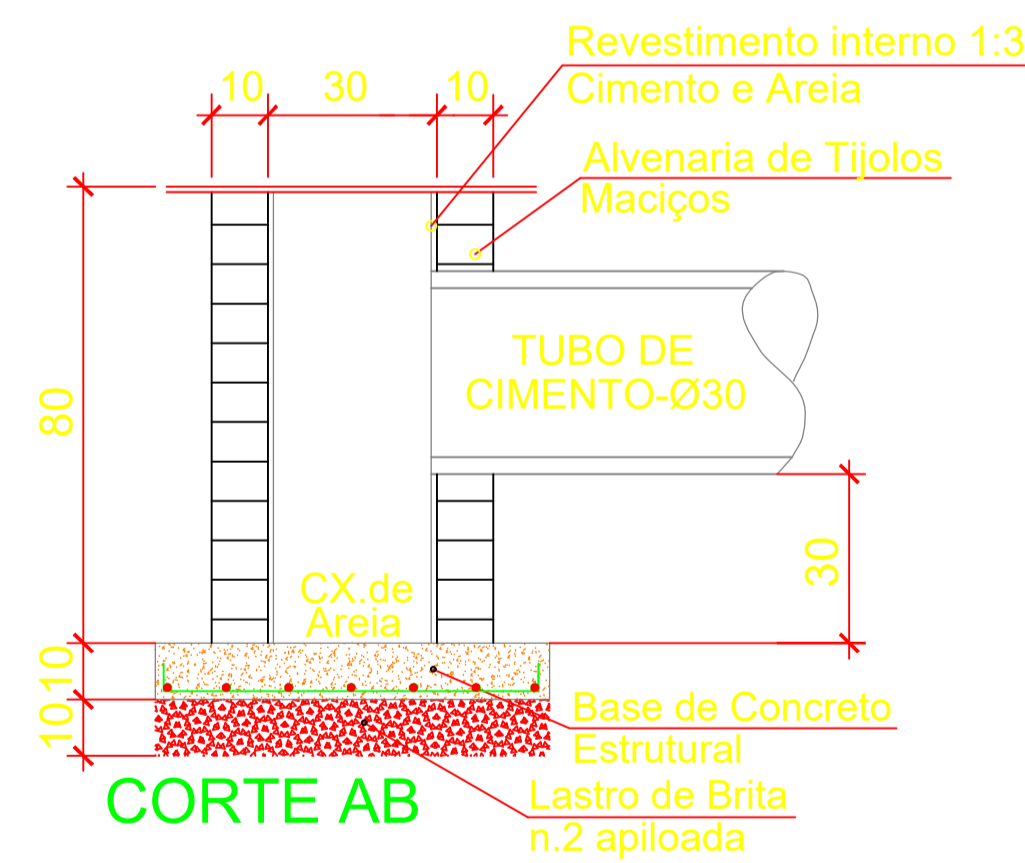
CORTE CD
