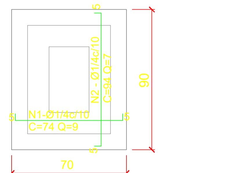
DETALHE LAJE DO FUNDO CONCRETO ESTRUTURAL
