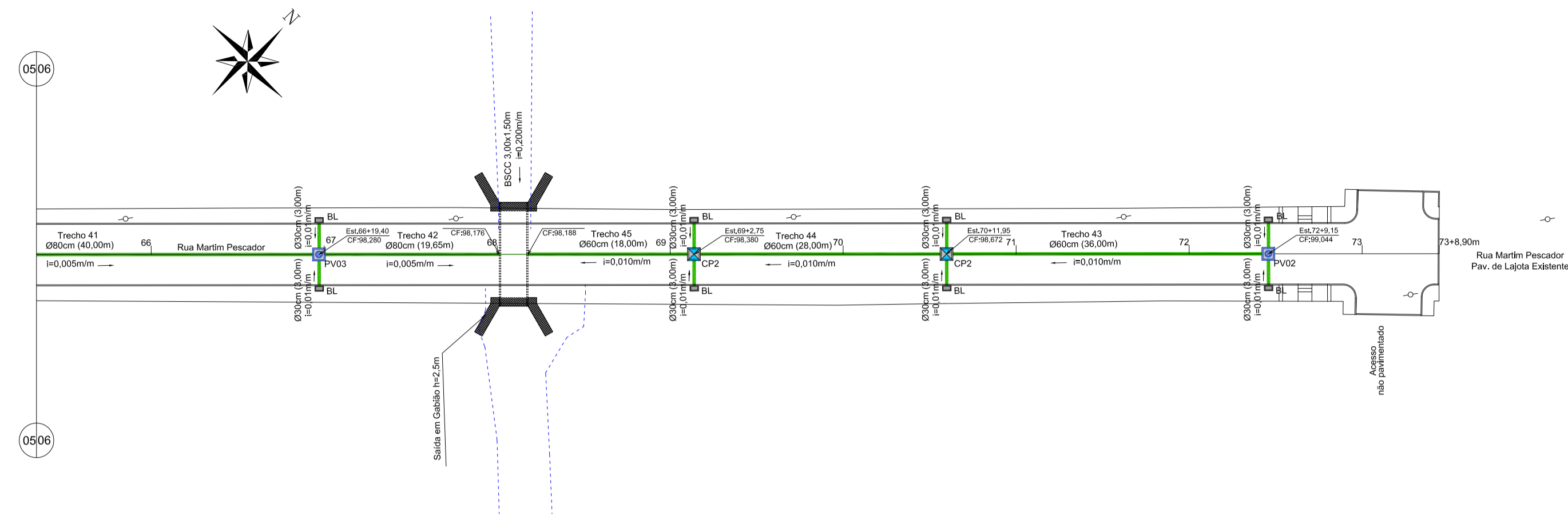
DRENAGEM PLUVIAL - Rua Martim Pescador - Articulação 06 Escala 1:500
