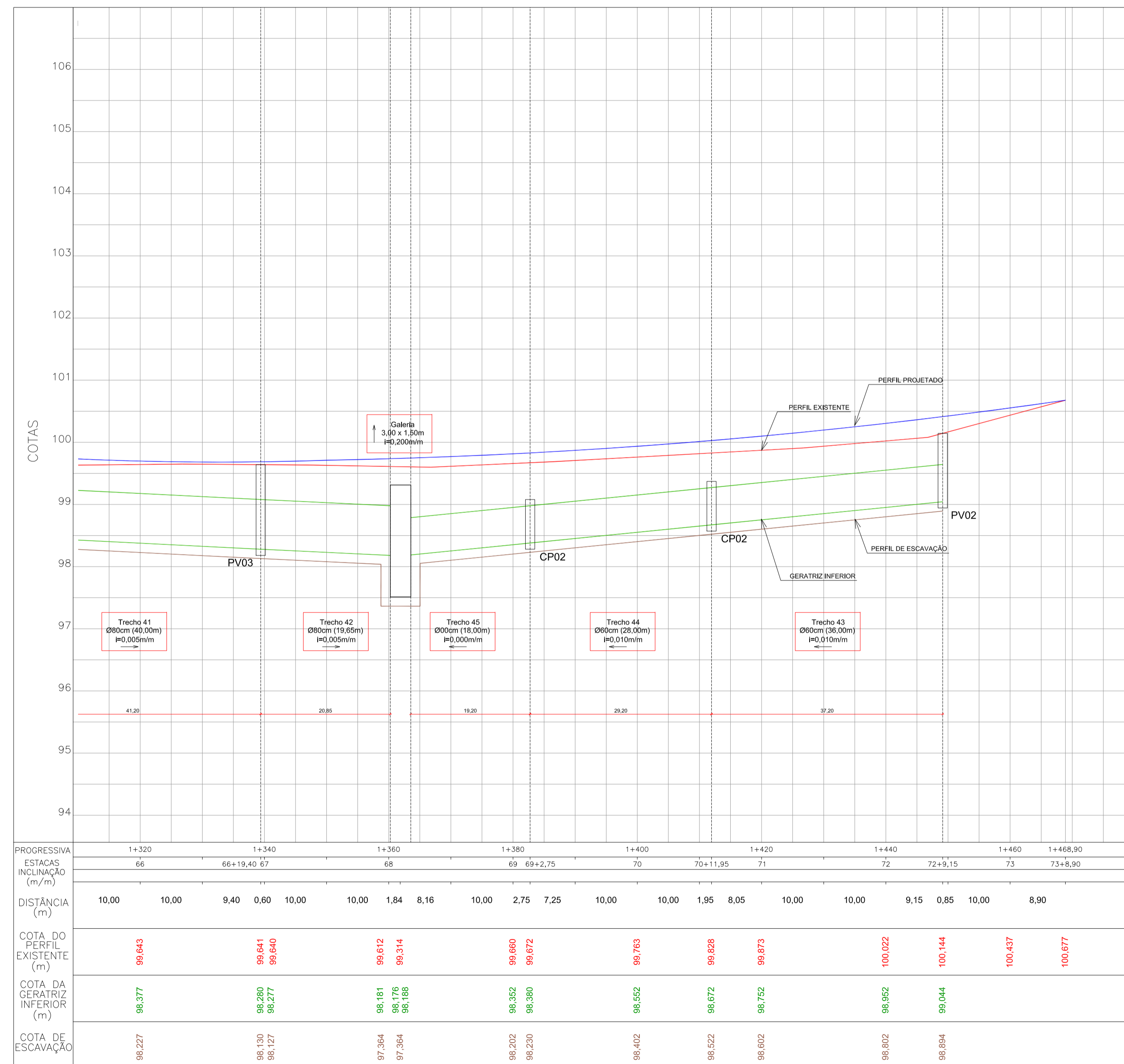
DRENAGEM PLUVIAL - Rua Martim Pescador - Articulação 06 Escala 1:500
